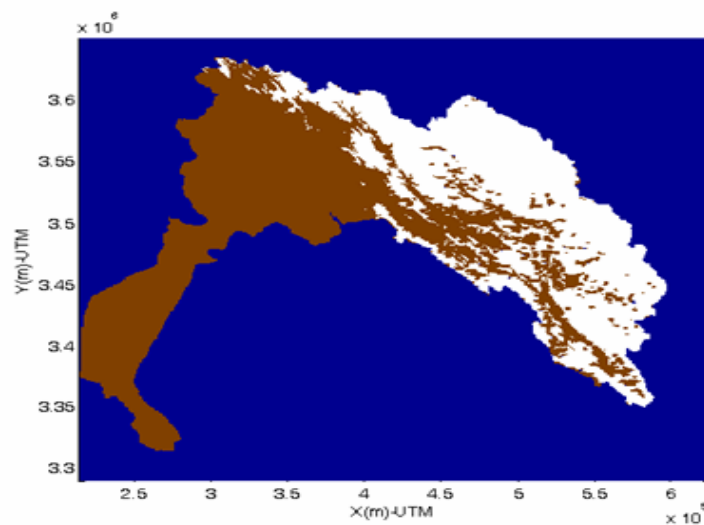
شكل (۲) سطح پوشش برف حوضه كارون بر اساس تصاوير MODIS در تاريخ ۲۰-۰۱-۲۰۰۱
