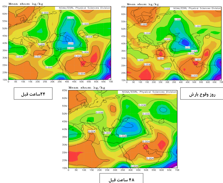
شکل (۱۷) نقشه میانگین تراز میانی جو در الگوی ششم
